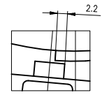
B 2:1 DETAIL POLOHY ROTORU VŮČI SNÍMAČI V OKAMŽIKU PŘESKOKU JISKRY PLATI PRO OTAČKY 4000 MIN -1
