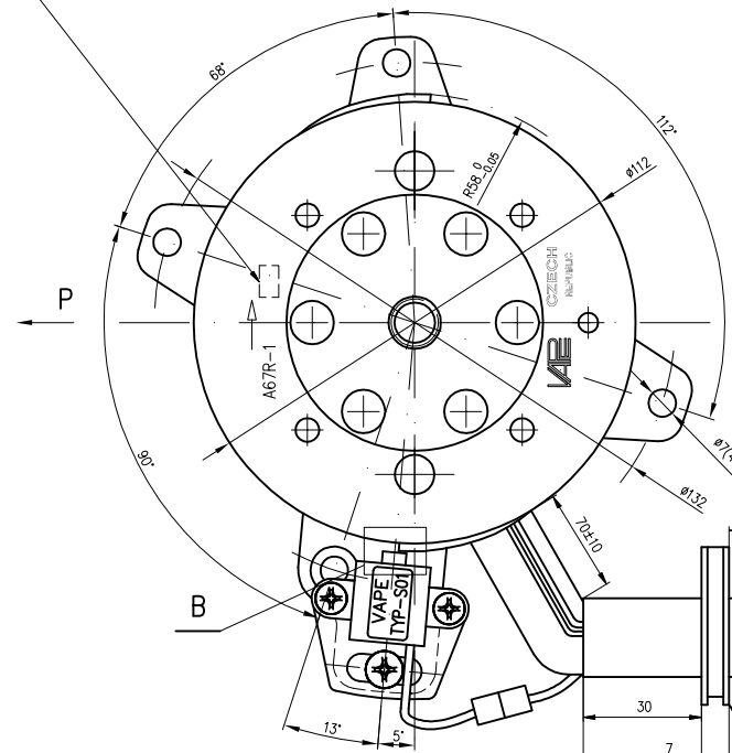
B 2:1 DETAIL POLOHY ROTORU VŮČI SNÍMAČI V OKAMŽIKU PŘESKOKU JISKRY PLATI PRO OTAČKY 4000 MIN -1
